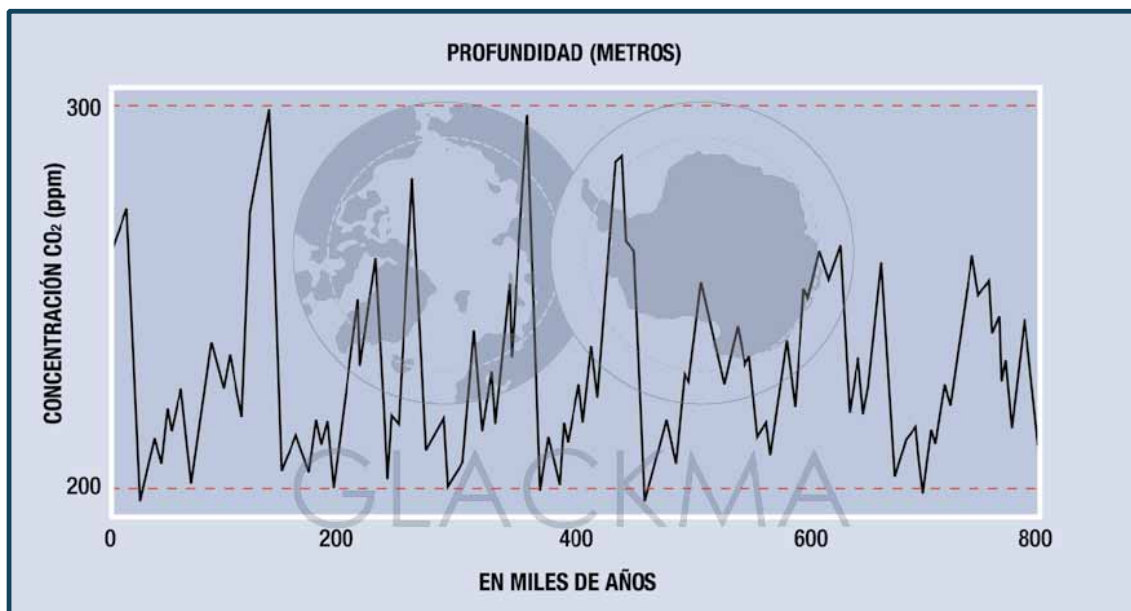
Registro en Domo C - Calendario anual de 800.000 años
