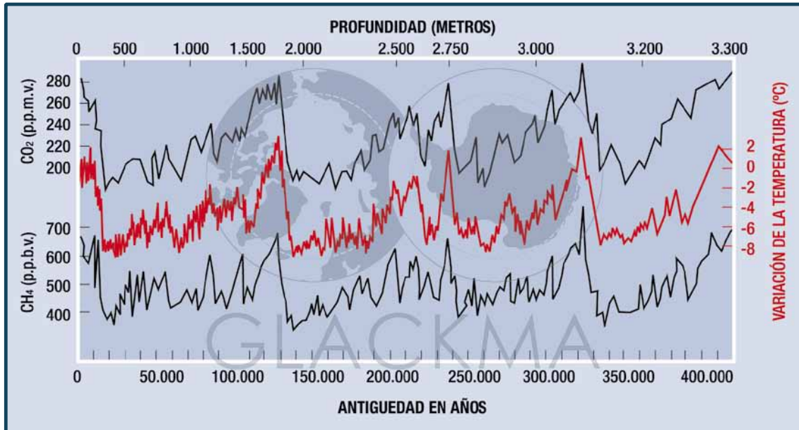
Registro en el hielo de Vostok - Distribución de CO 2 , CH 4 y paleotemperatura de 420 000 años
