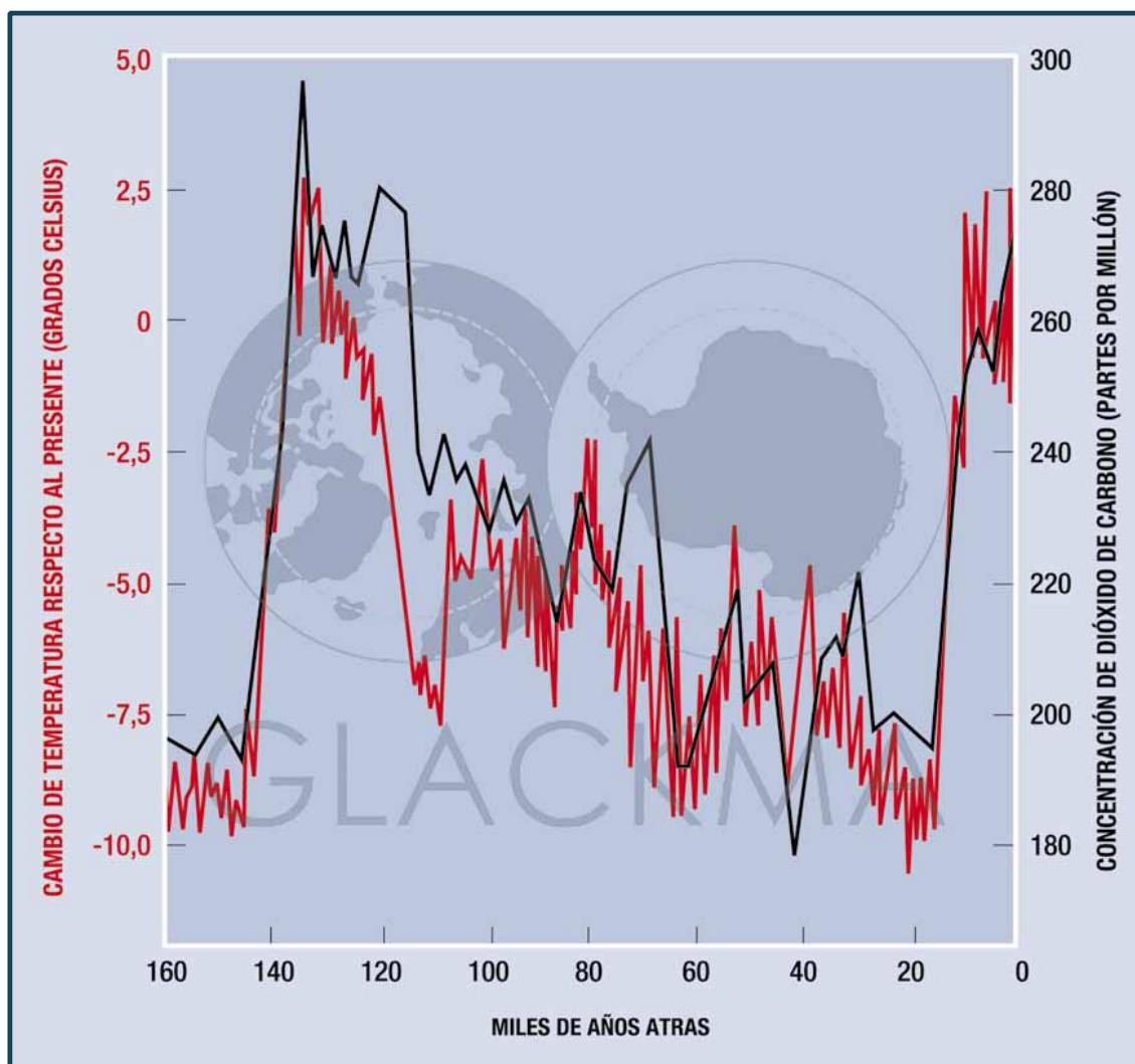
CO 2 y paleotemperatura en los últimos 160.000 años
