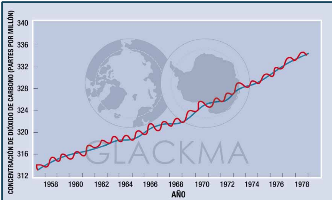
Registro continuo de CO 2 en el Polo Sur (Antartida)
