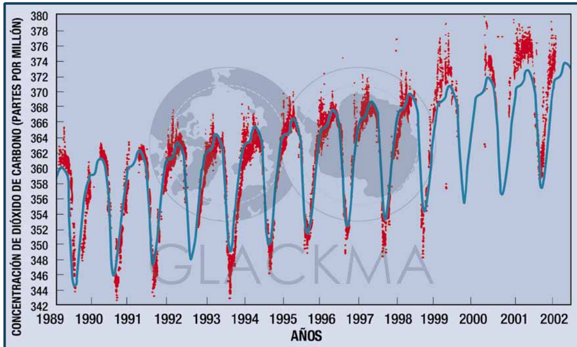
Registro continuo de CO 2 en Ny-Alesund (Ártico)
